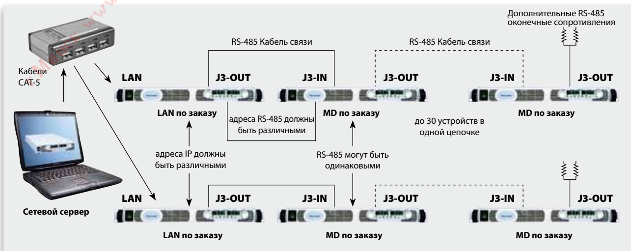
Конфигурация многоканального интерфейса системы источников питания
