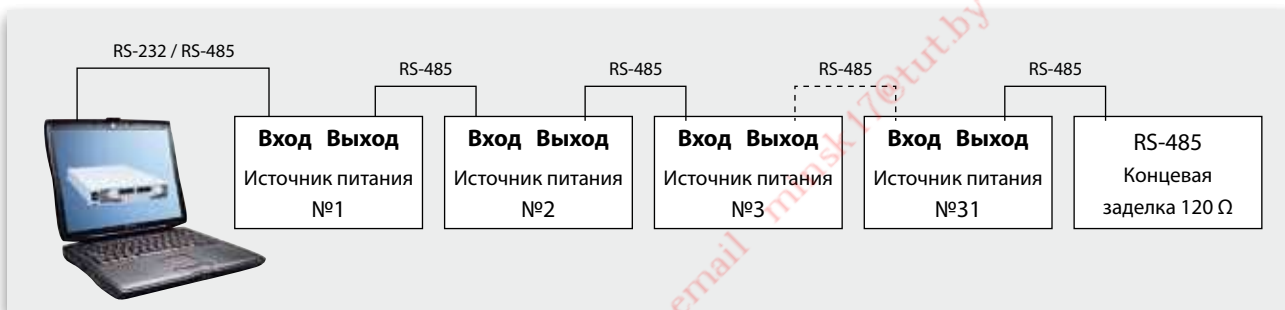
Связь по интерфейсу RS-232 / RS-485 между несколькими источниками питания
