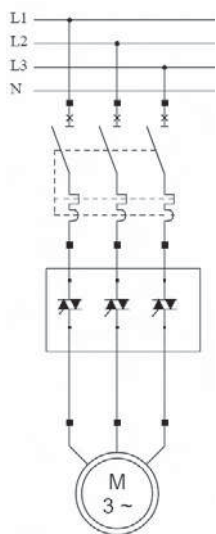
Трехфазное ТТП SVT8/SGT8, управляющее трехфазным двигателем, с термомангнитной защитой
