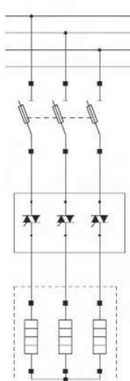
Трехфазное ТТП SCT/SVT/SGT для управления нагревательными элементами, соединенными звездой, с предохранителями
