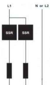
2 регулятора нагрузки, одна фаза
