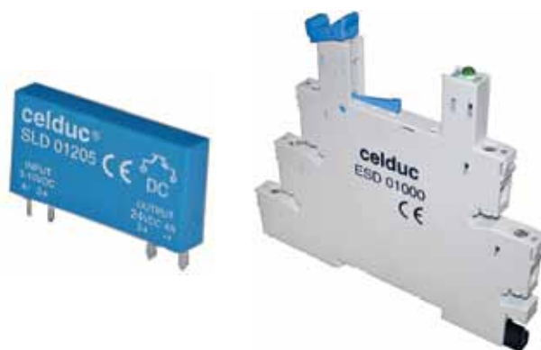
Рис.3. ТТР серии SLIM и кронштейн для его установки на DIN-рейку
