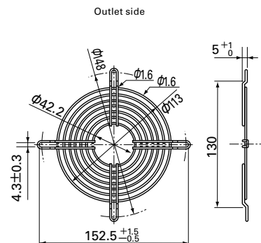
Mass : 32g
