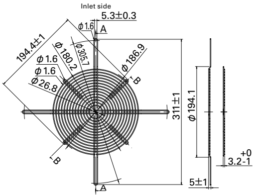
Mass : 106g
