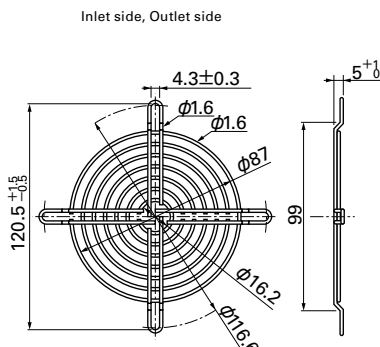
Mass : 29g
