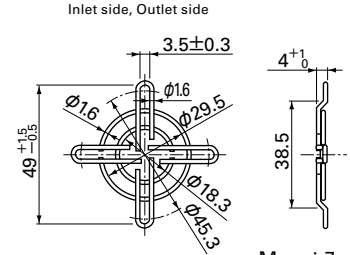
Mass : 7g
