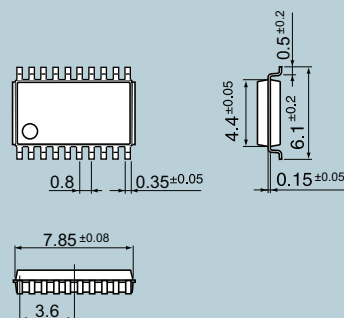
SSOP-20
