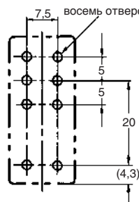
Крепежные отверстия
