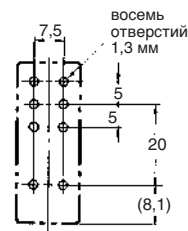
Крепежные отверстия
