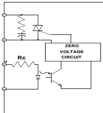
AC OUTPUT
